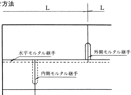
側面
