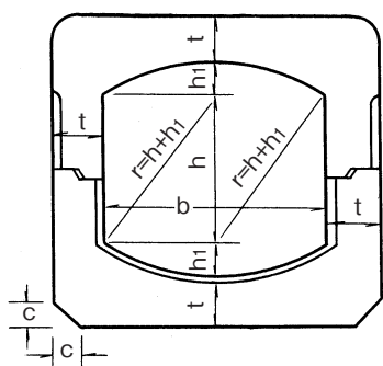
断面
