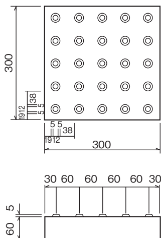
SM300-JB-60
