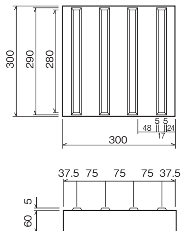
SM300-JC-60
